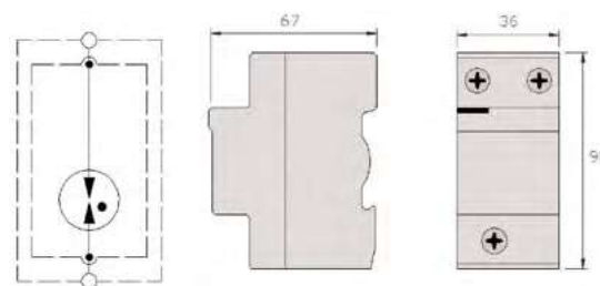
Esquema y dimensiones del AD1-200/240
