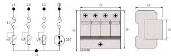
Esquema y dimensiones del BD4-60
