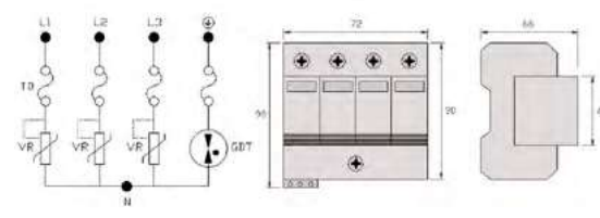
Esquema y dimensiones del BD4M-50/240
