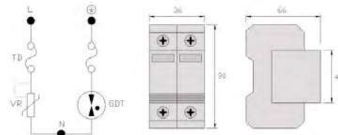
Esquema y dimensiones del BD2-60
